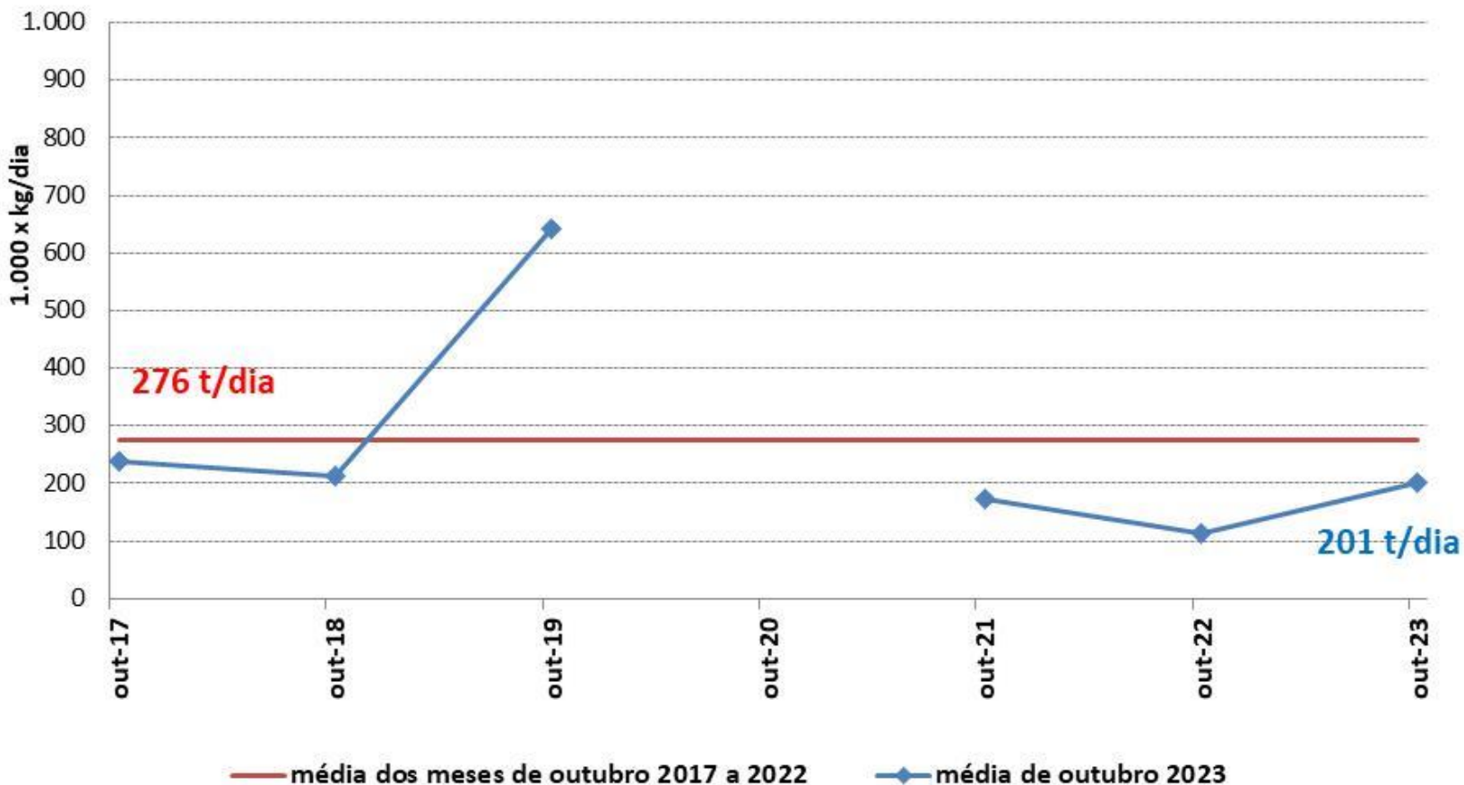
Carga de Matéria Orgânica - OUTUBRO Exutórios do Tietê e Pinheiros
