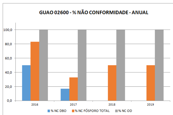
Figura 5 – Percentual de não conformidade – GUAO 02600.
