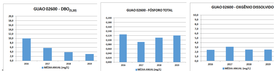
Figura 4 – Concentração de DBO (5,20) , Fósforo Total e Oxigênio Dissolvido – GUAO 02600.
