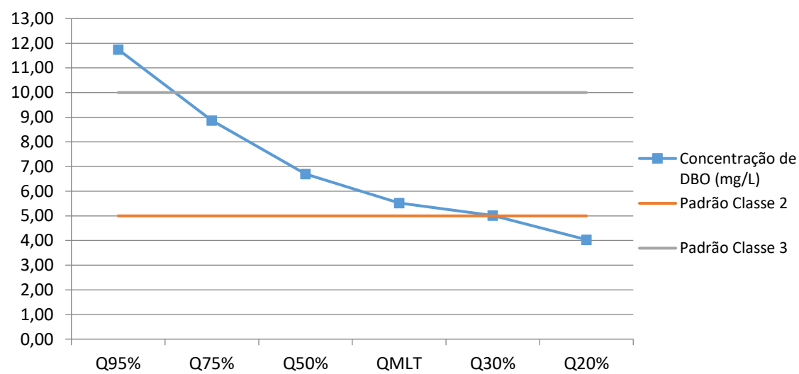
Figura 3 – Correlação da concentração de DBO X vazão de referência na captação.
