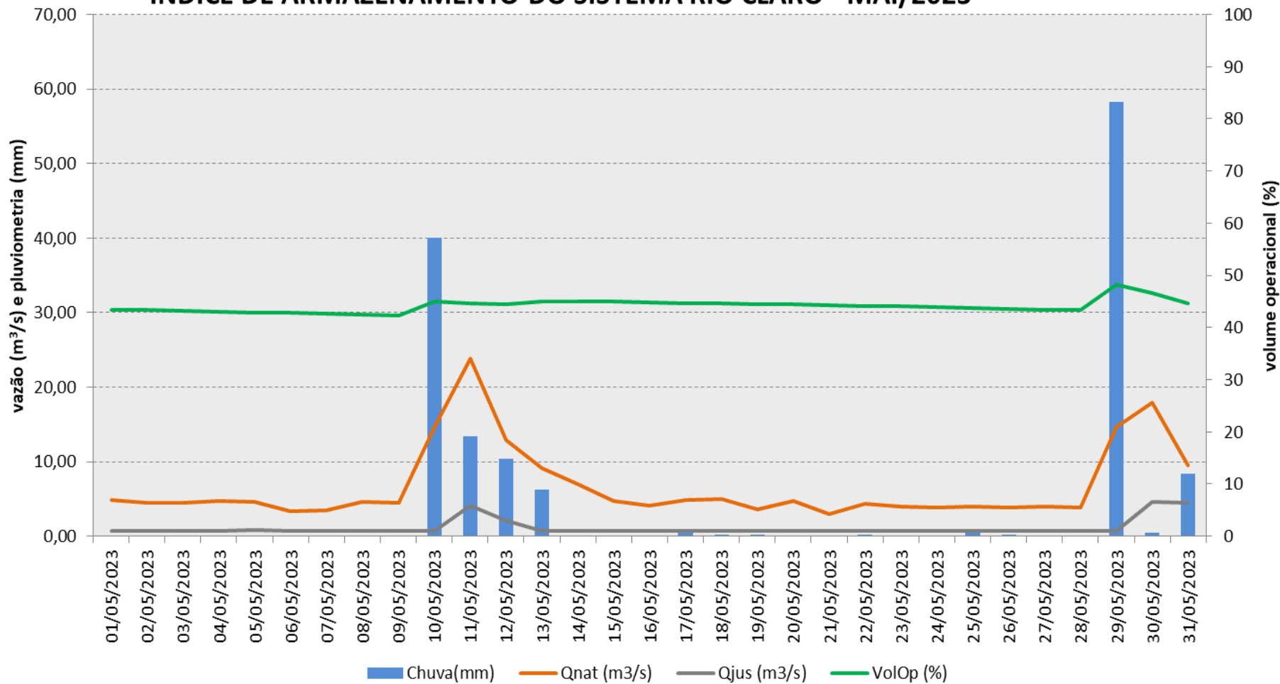
ÍNDICE DE ARMAZENAMENTO DO SISTEMA RIO CLARO - MAI/2023
