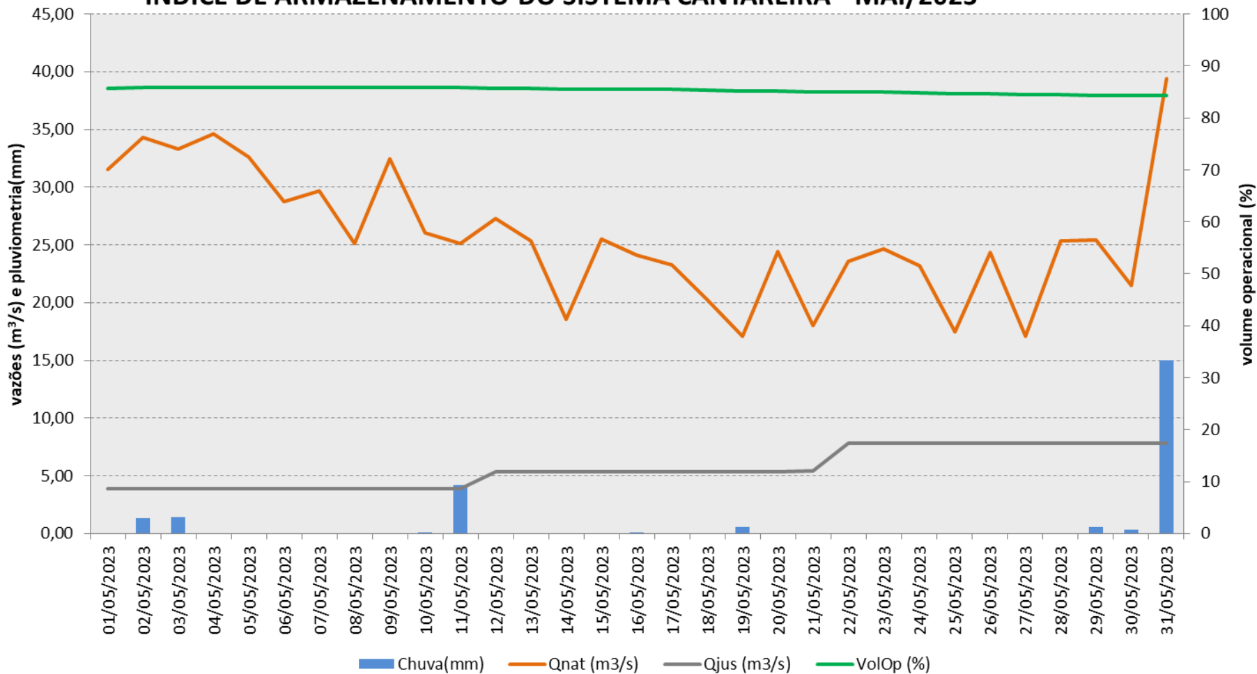
ÍNDICE DE ARMAZENAMENTO DO SISTEMA CANTAREIRA - MAI/2023
