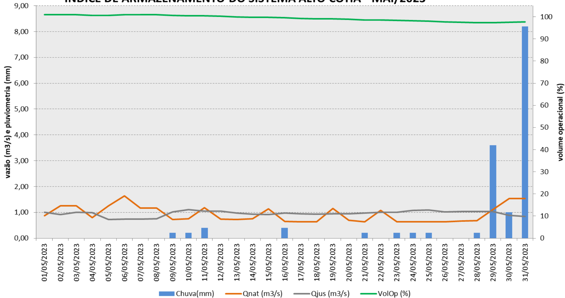
ÍNDICE DE ARMAZENAMENTO DO SISTEMA ALTO COTIA - MAI/2023
