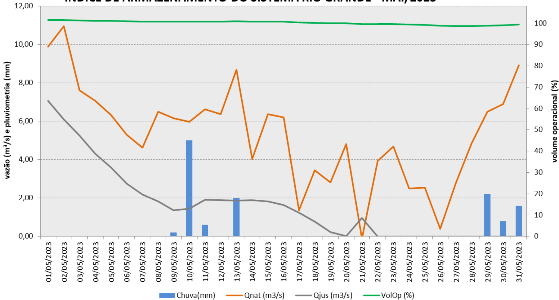
ÍNDICE DE ARMAZENAMENTO DO SISTEMA RIO GRANDE - MAI/2023
