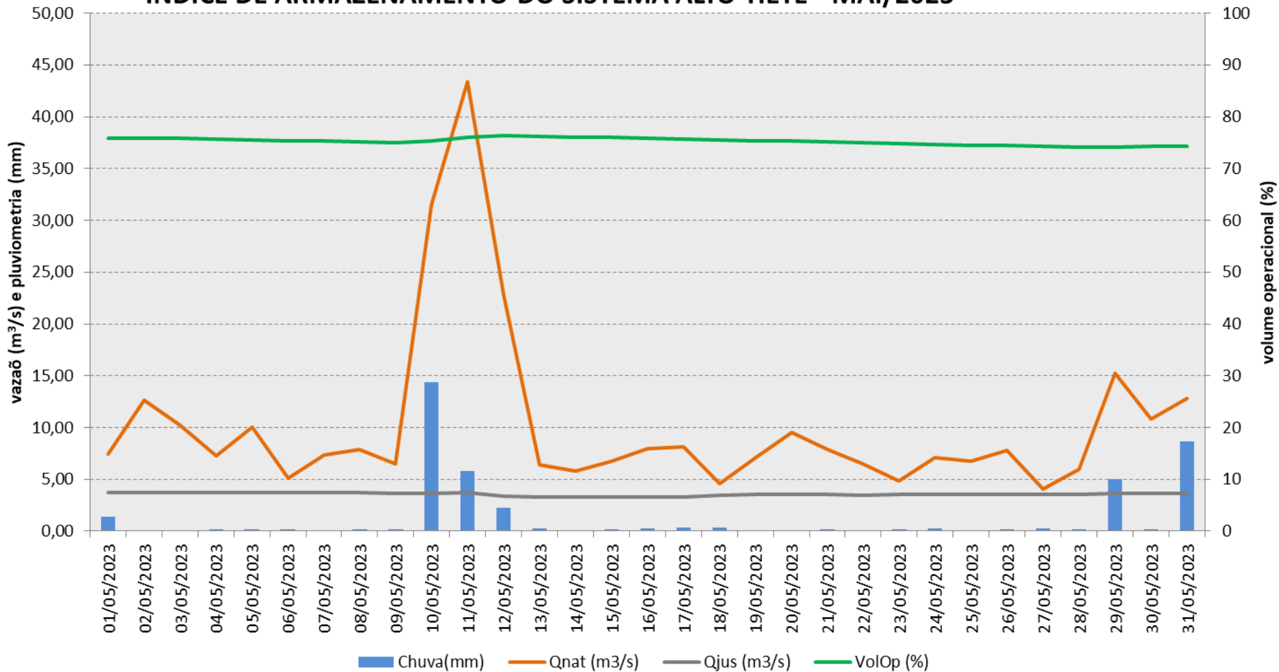
ÍNDICE DE ARMAZENAMENTO DO SISTEMA ALTO TIETÊ - MAI/2023
