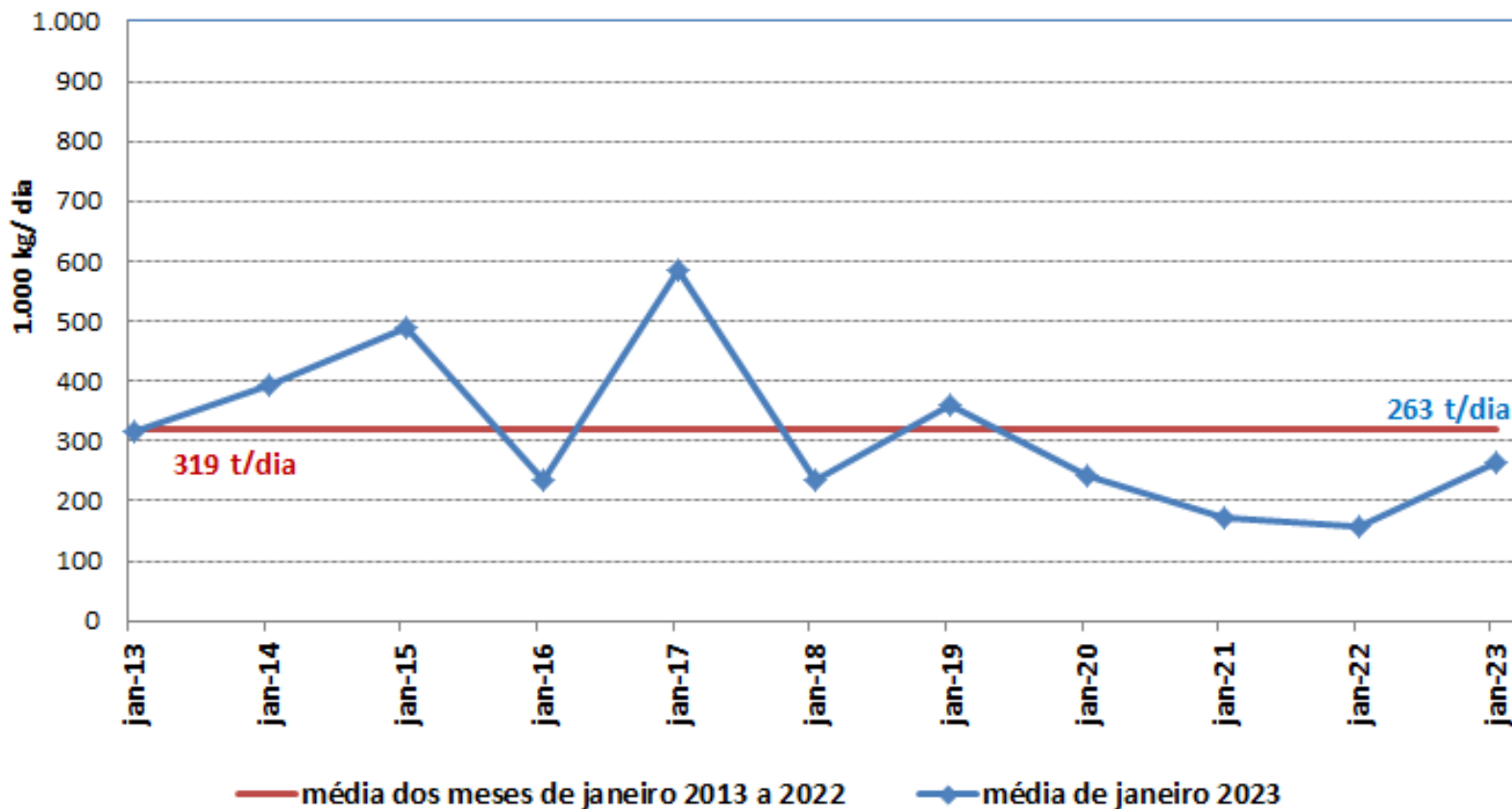
Carga de Matéria Orgânica - JANEIRO Exutórios do Tietê e Pinheiros
