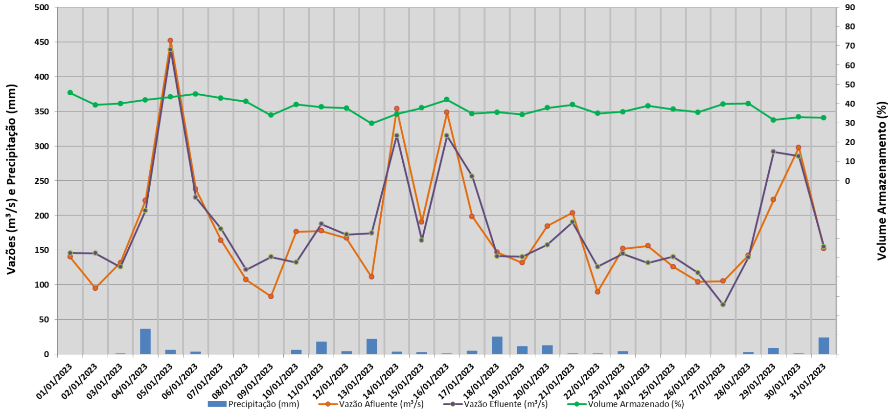
Reservatório de Pirapora - Janeiro/2023
