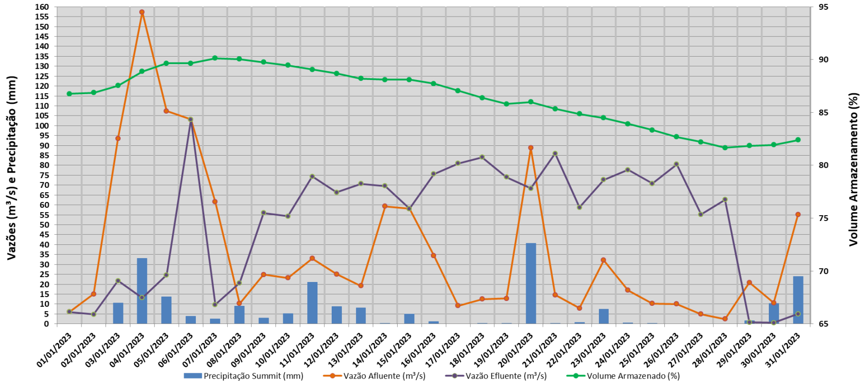
Reservatório Billings (Compartimento Pedreira) - Janeiro/2023
