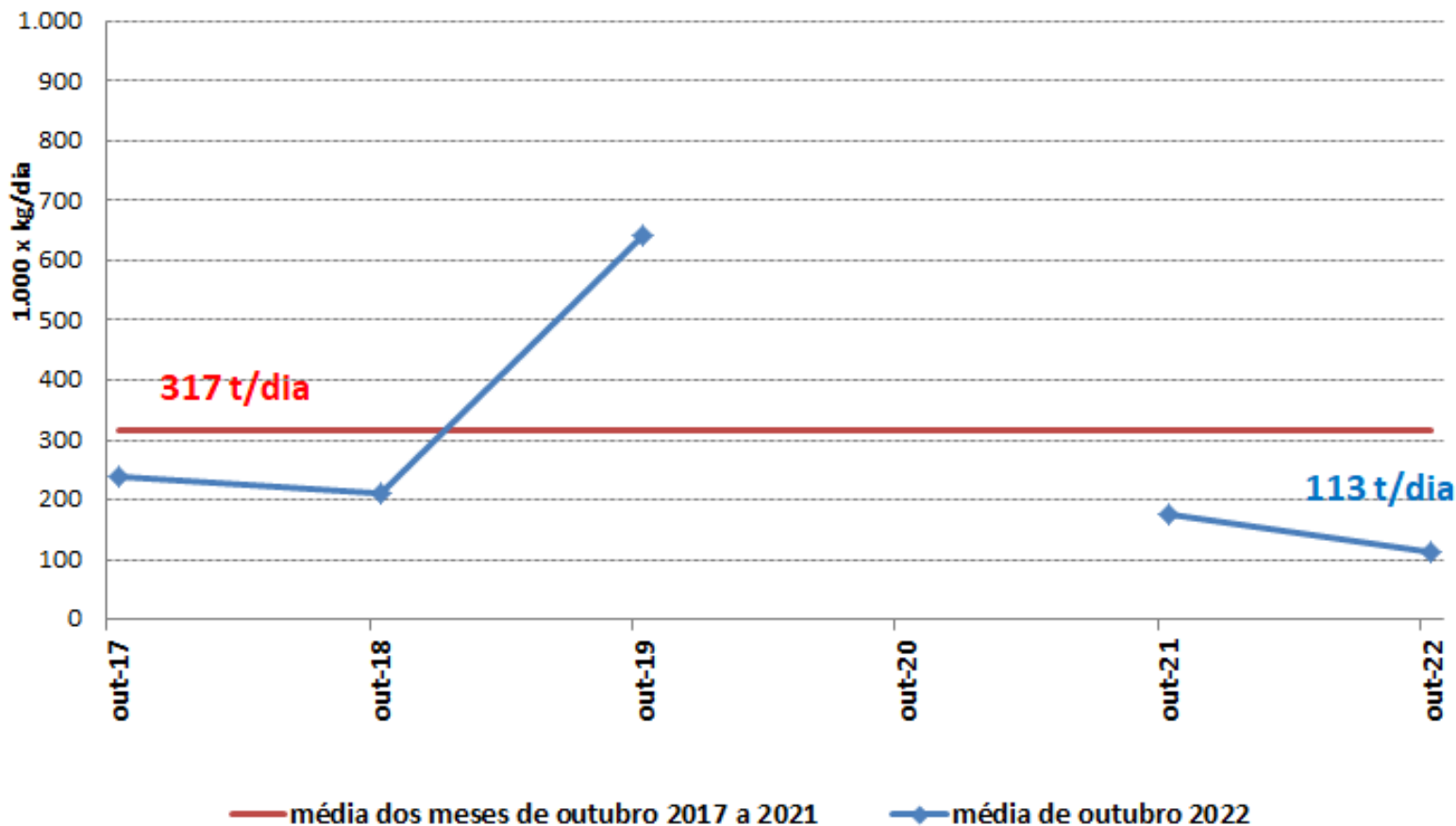
Carga de Matéria Orgânica - OUTUBRO Exutórios do Tietê e Pinheiros
