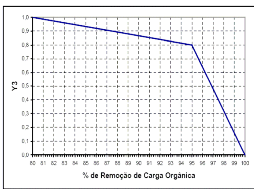
Gráfico de Remoção de Carga Orgânica
